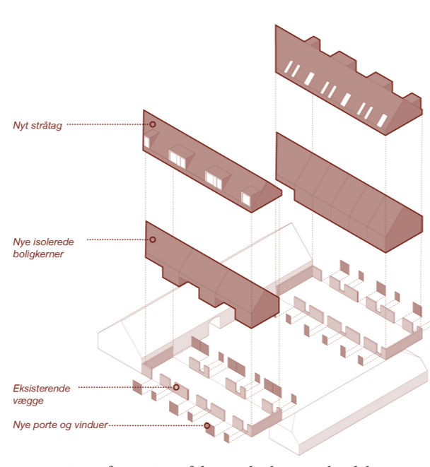
Isometri/ transformation af de mindre længer, der delvist fores med isolerende kerner og nye vinduesåbninger i tag og facade.
