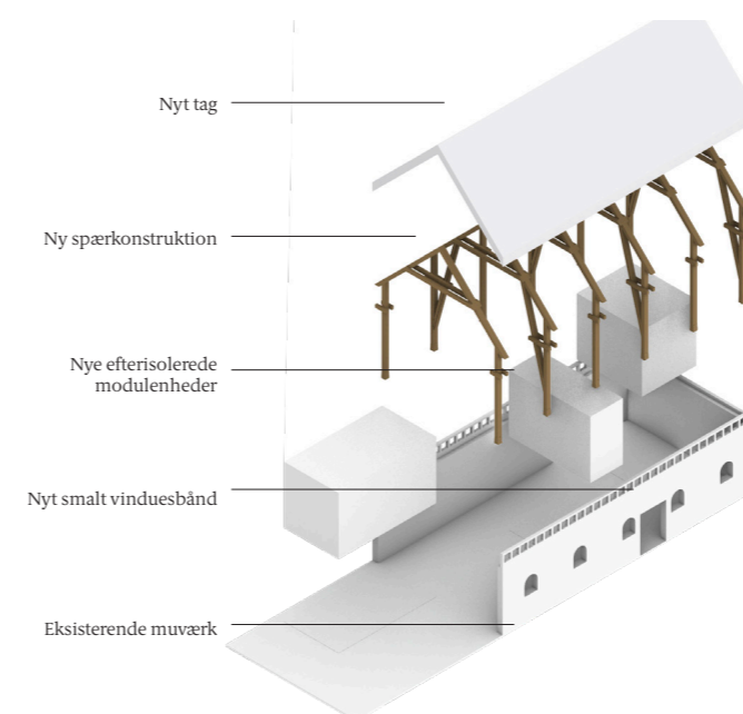
Princip for transformation af en lade. Muværk bevares og ladens inde fores med isolerende modulenheder.
